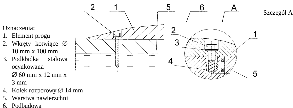
Rys. 4. Przykład umocowania progu do nawierzchni jezdni
