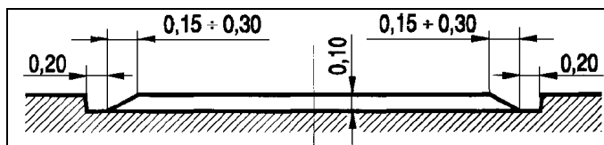
Rys. 5. Przekrój poprzeczny progu zwalniającego liniowego o zmniejszonej szerokości (progów skróconego) w przekroju poprzecznym jezdni
