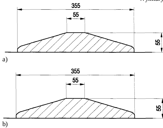
KSZTAŁT I WYMIARY W PRZEKROJU POPRZECZNYM PRZYKŁADOWYCH PROGÓW PODRZUTOWYCH (wg [23]) Wymiary w mm
