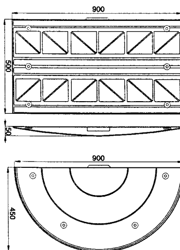
Rys. 3. Próg typu listowego długości 900 mm i wysokości 50 mm
