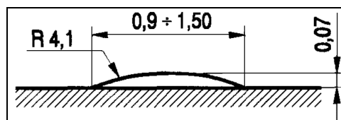
Rys. 5. Przekrój poprzeczny progu zwalniającego liniowego o zmniejszonej szerokości (progów skróconego) w przekroju poprzecznym jezdni
